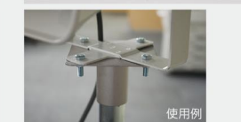
396-51 (AC100V用) サイズ:62×100×100 材質:鉄(メタリックグレー塗装仕上げ)
